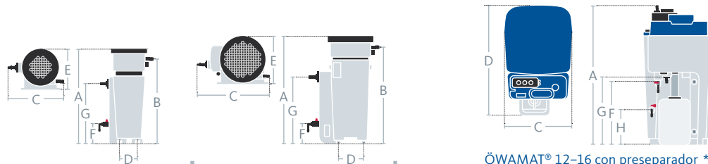
ÖWAMAT® 12-16 con preseparator *
